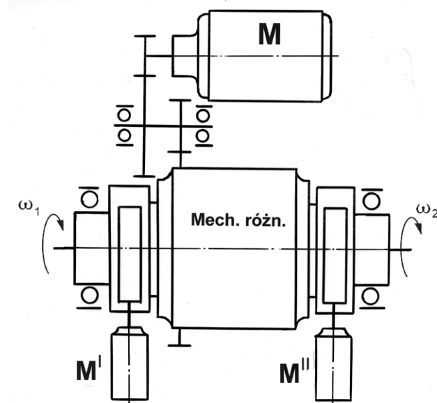
Rys. 7. Konceptcja autora elektryczno-mechanicznego systemu kierunkowego napędzania pojazdu
