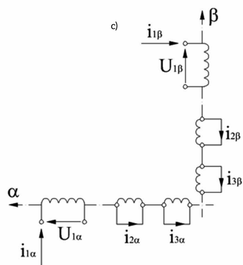
Rys. 2. Kolejne etapy transformacji uzwojeń silnika indukcyjnego klatkowego z układu trójfazowego do układu dwuosiowego \alpha, \beta : a – przekrój obwodu magnetycznego; b – schematyczne przedstawienie uzwojeń; c – uzwojenia w osiach \alpha, \beta nieruchomych względem stojana
