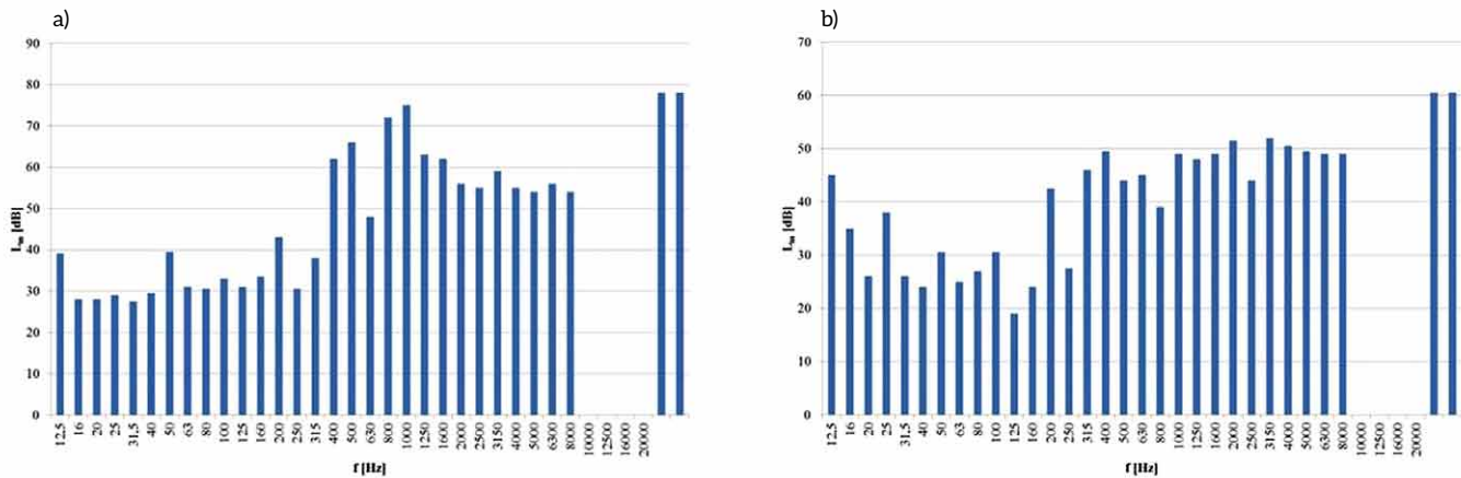
Rys. 11. Widmo tercjowe hałas mikrozasilacza: a) przed modernizacją (praca niestabilna), b) po modernizacji (praca stabilna) [7]
