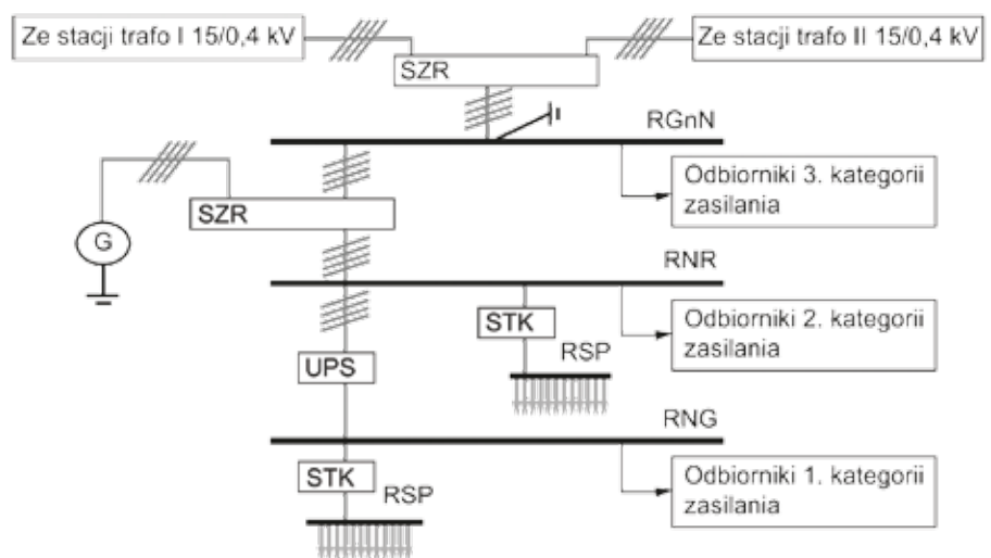
Rysunek 2.1. Uproszczony schemat instalacji zasilającej inteligentnego budynku. Legenda: SZR – Samoczynne Załączenie Rezerwy; STK – Siłownia Telekomunikacyjna; UPS – zasilacz bezprzerwowo; G – generator prądotwórczy; RGnN – rozdzielnia główna niskiego napięcia; RNR – Rozdzielnia Napięcia Rezerwowego; RNG – Rozdzielnia Napięcia Gwarantowanego; RSP – Rozdzielnia Stałoprądowa 48 V
