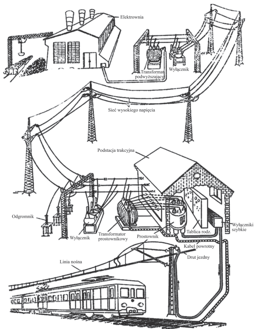
Rys. 2. Poglądowy schemat zasilania w energię kolei elektrycznej korzystającej z sieci trakcyjnej prądu stałego. Źródło: [A4]
