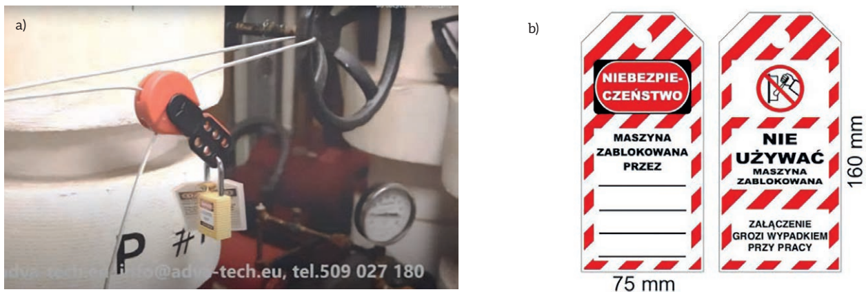
Rys. 1. Urządzenia do blokowania i oznaczania: blokada linkowa: a) przód; b) etykieta
