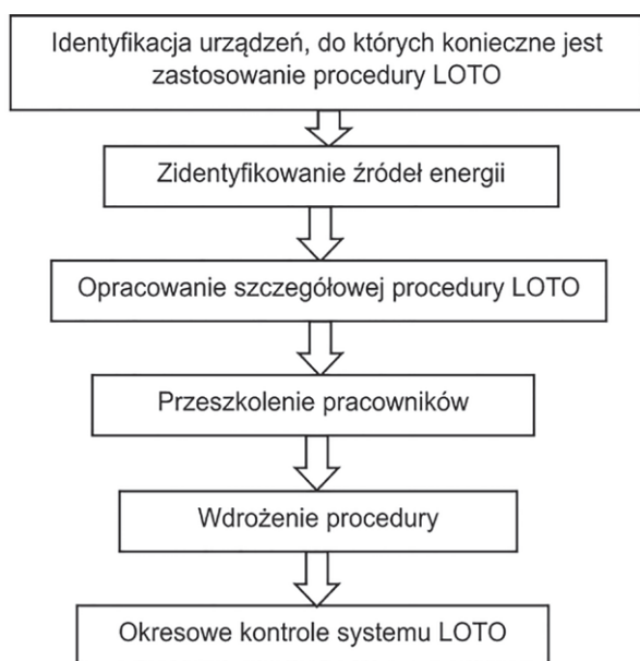
Rys. 2. Ogólna procedura postępowania przy wdrażaniu LOTO
