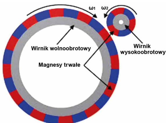
Rys. 3. Przekładnia magnetyczna modelująca przekładnię mechaniczną [3, 4]
