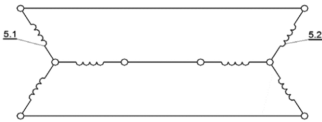
Rys. 5. Schemat połączenia uzwojeń przy pracy jednokierunkowej przekładni
