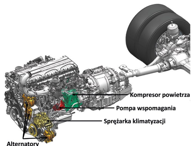
Rys. 5. Akcesoria zasilane z silnika spalinowego [1]
