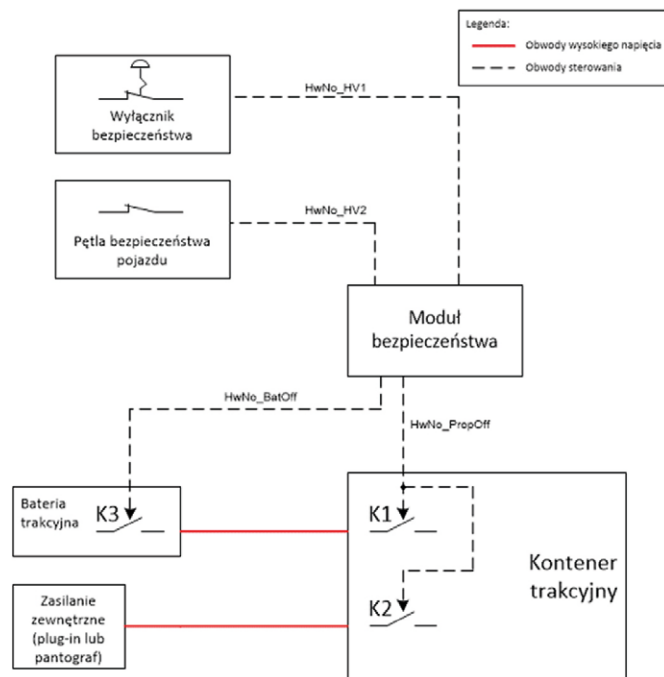
Rys. 10. Wyłącznik awaryjny i pętla bezpieczeństwa [1]
