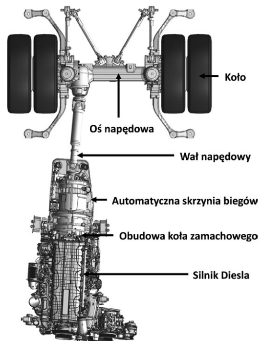
Rys. 4. Architektura systemu napędowego - napęd konwencjonalny [1]
