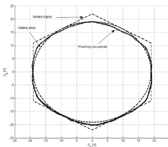
Rys. 4. Przebieg sinusoidalnej, trapezoidalnej oraz rzeczywistej siły elektromotorycznej w układzie \alpha - \beta dla rowerowego silnika bezprzekładniowego
